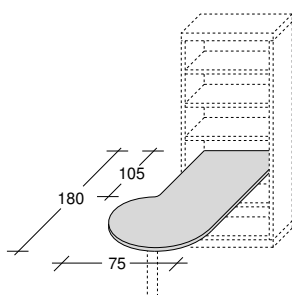
per colonna GLOBO L. 60 cm. for coloumn GLOBO L. 60 cm
